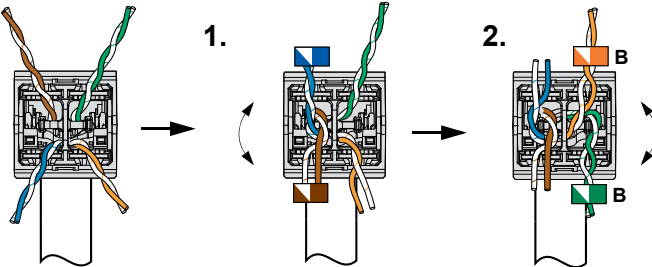
Cable End 2
