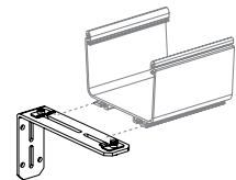
FR6LB – Soporte QuikLock™ en "L" de Montaje en Muro
