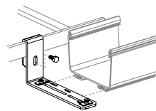
FR6LRB – Soporte de Escalera Portacables
